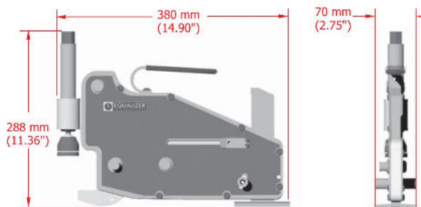
Tool dimensions
