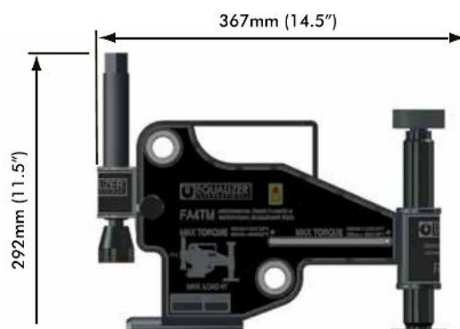
Tool dimensions
