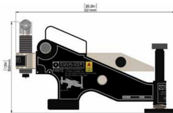
Tool dimensions
